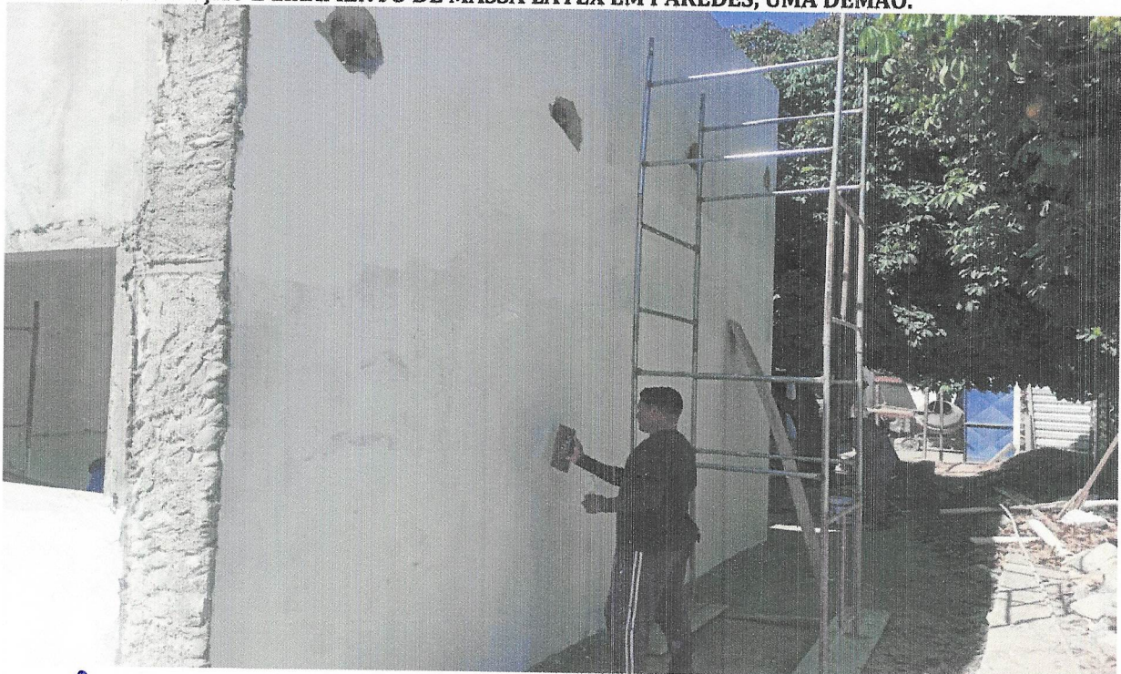
FOTO 12 - APLICAÇÃO E LIXAMENTO DE MASSA LÁTEX EM PAREDES, UMA DEMÃO.
