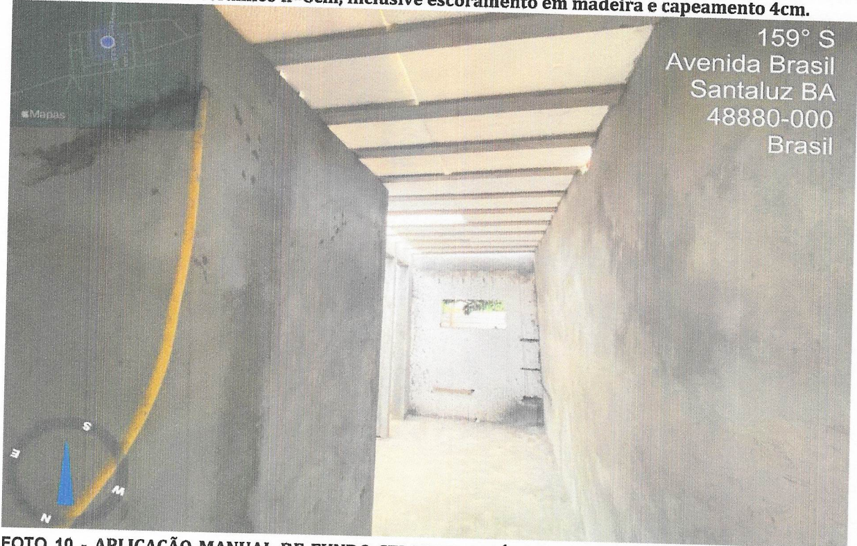
FOTO 10 - APLICAÇÃO MANUAL DE FUNDO SELADOR ACRÍLICO EM PAREDES EXTERNAS DE CASAS. AF_06/2014
