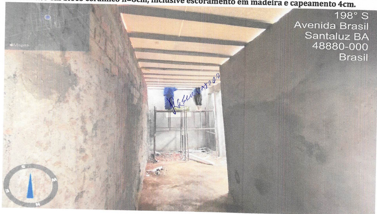
FOTO 08 - Laje pré-fabricada treliçada com vigota dupla para piso, intereixo 38cm, h=12cm, enchimento em bloco cerâmico h=8cm, inclusive escoramento em madeira e capeamento 4cm.
